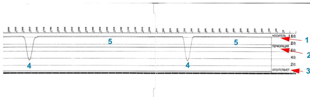
Рис.5 • Профиль датчика (носитель с черными метками)
